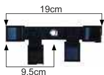
Faja de fijación 4 puntos para sillas de ruedas 25mm 25mm 4 points fixing strap for wheelchairs 99 75 FX 4P CD
